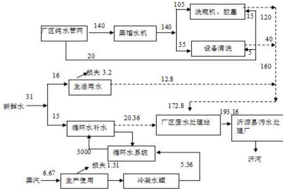
图3 项目水平衡图 单位：m³/d
