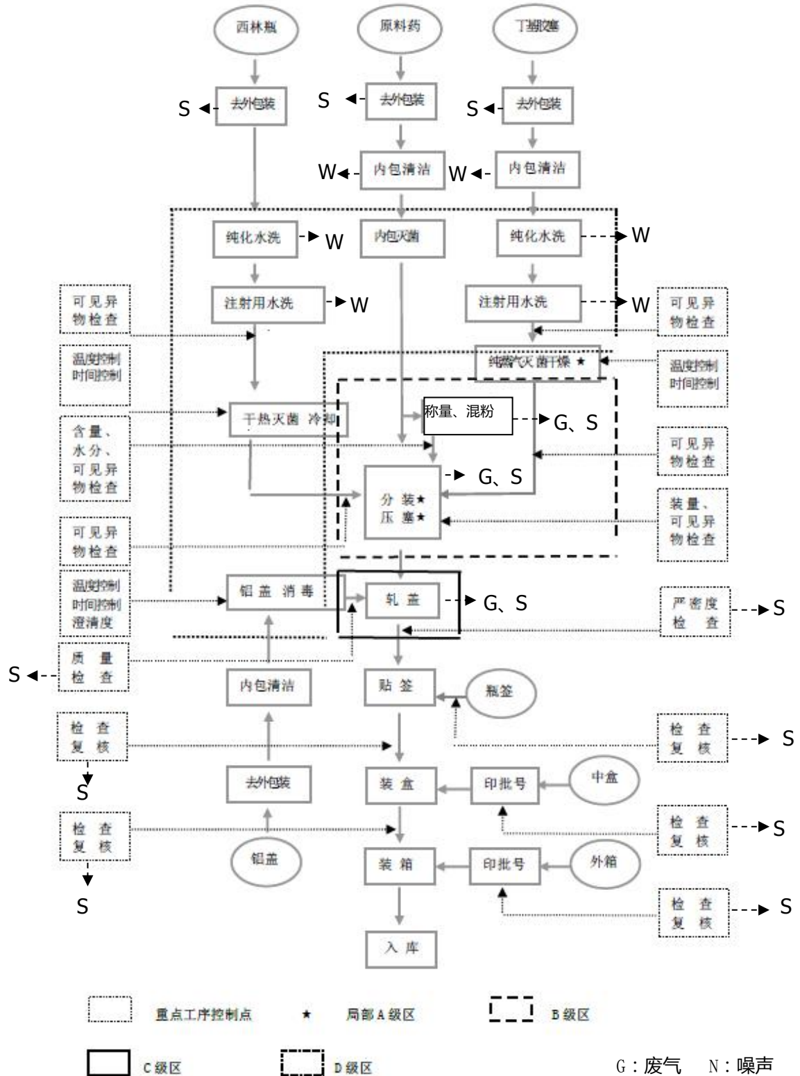
图4 项目生产工艺流程及产污环节图
